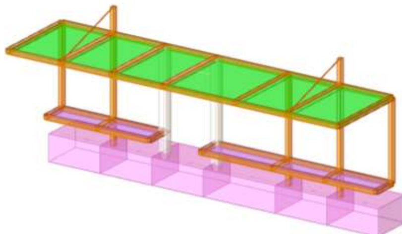
Figura 2. Vista 3D del modello geometrico
